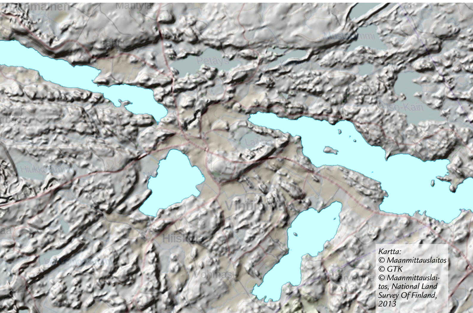
Vihtijärven korkokartta. Kuvassa nähdään hyvin alueen maisemarakenne eli laaksot, vesistöt, selänteet ja harjumuodostelmat. Alla Vihtijärven keskustan kallioperäkartta.
